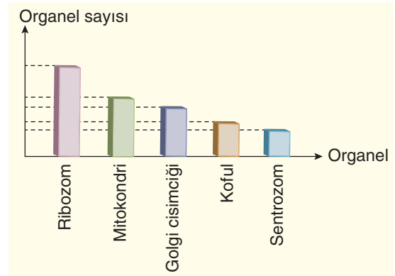
Hücre II
